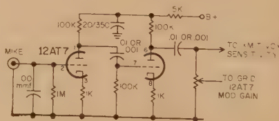
Fig. 2—Original SB-10 input circuit.
