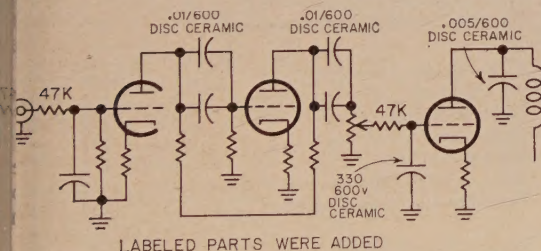
Fig. 6—SB-10 modifications.
