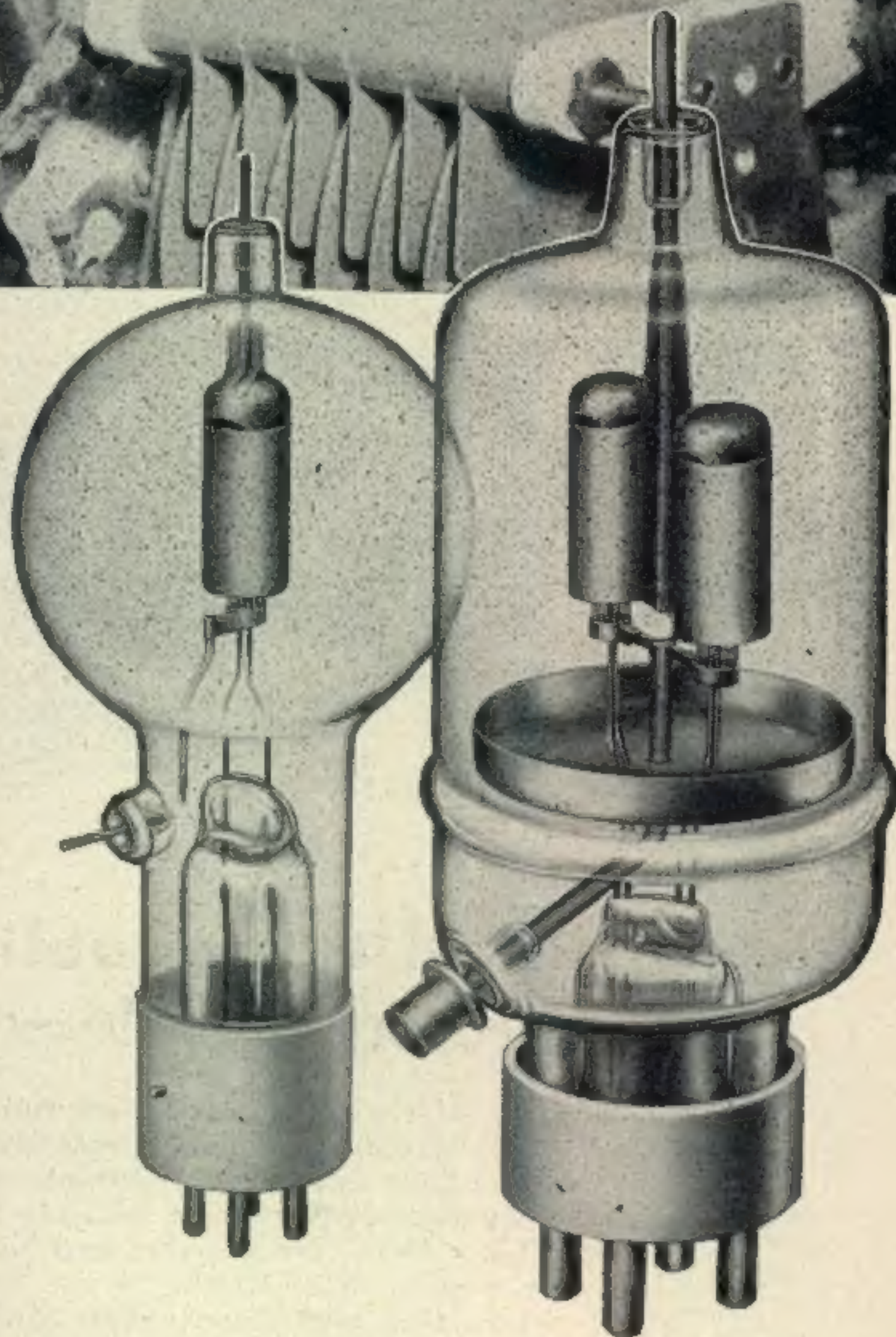
EIMAC 75T POWER TRIODE
